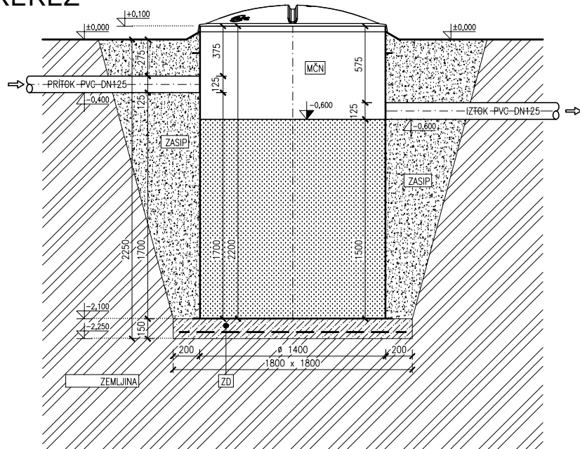
PREREZ
